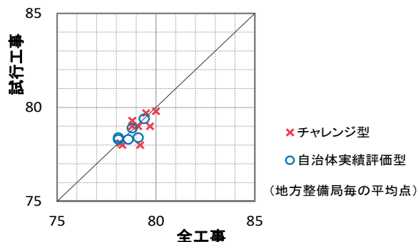
図-2 工事成績の比較（チャレンジ型等）
