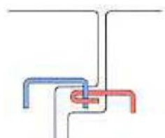
図-1 壁ブロックタイプ仮設車両用防護柵のブロック間の連結構造の例 2)
