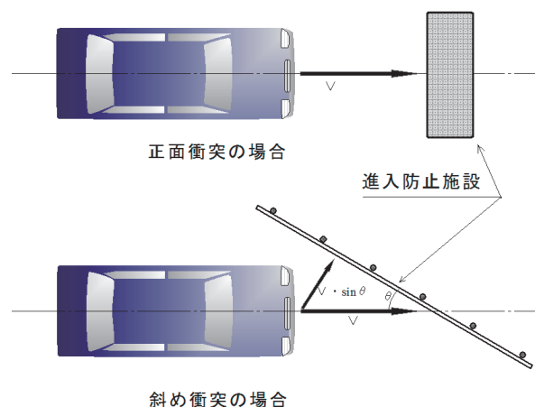
図-2 車両進入時の設計衝突速度の考え方
