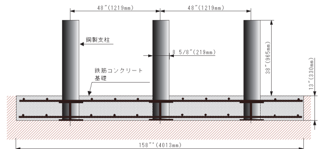
図-2 車両激突対応型ボラード(埋込み式)の製品例
