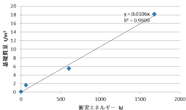
図-9 衝突エネルギーと基礎質量との関係
