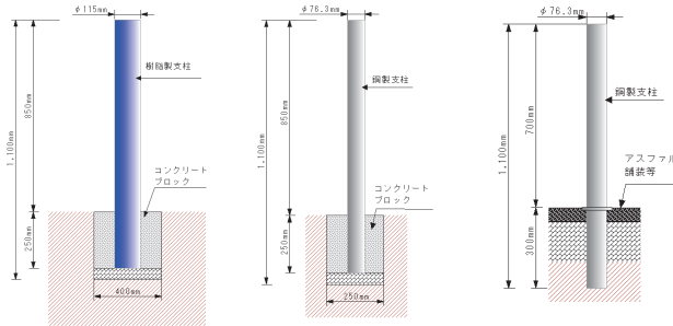
ブロック基礎構造 ブロック基礎構造 アスファルト舗装 (400×400×250) (250×250×250) 埋込み
