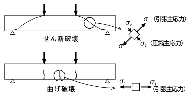
図-1 破壊の形態
