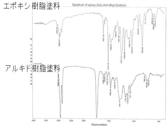
図-4 FT-IRを用いた塗膜の種類の見分け
