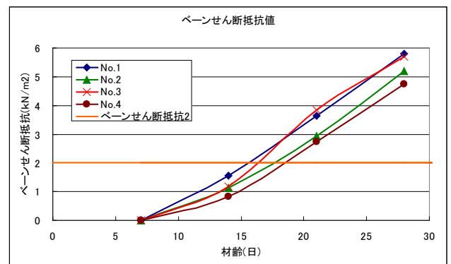
図-5 袋詰め底質の強度の発現状況
