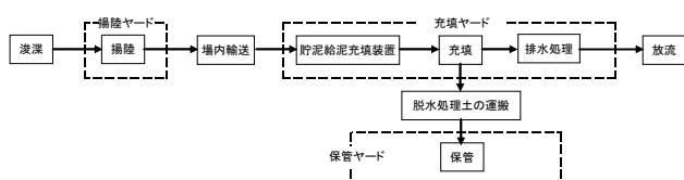
図-2 試験施工フロー
