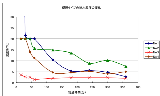
図-6 排水濁度の経時変化
