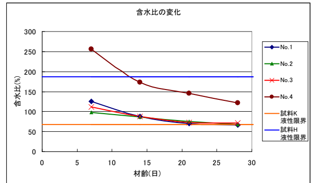
図-4 袋詰め底質の含水比の変化
