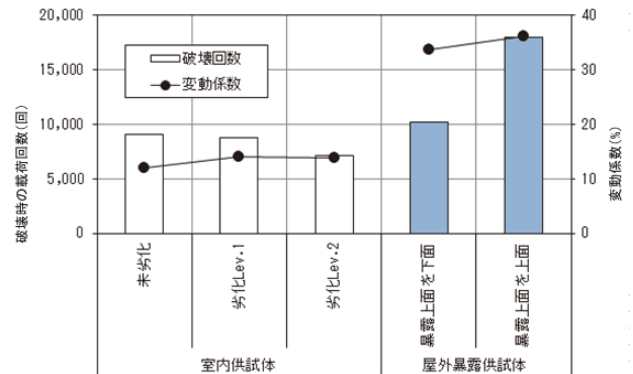
図-5 暴露供試体による曲げ疲労試験結果
