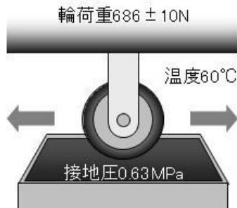
図-1 ホイールトラッキング試験の概略図
