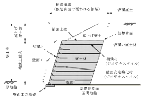
図-2 補強土壁の各部の名称
