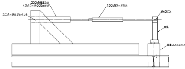
図-4 載荷方法
