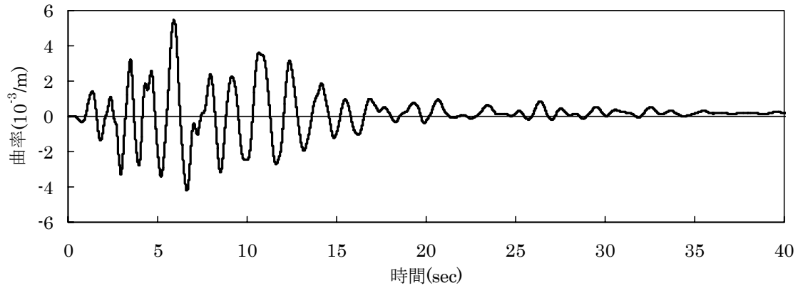
図-2.31 曲率 \phi の時刻歴応答波形の例
